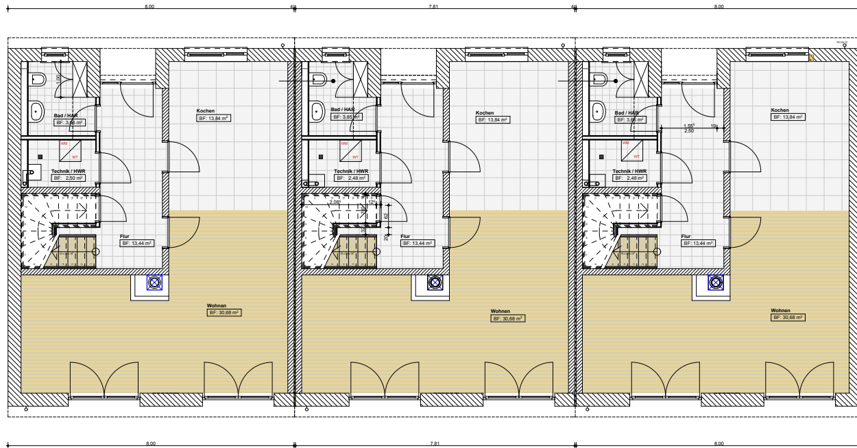
ERDGESCHOSS ENDHAUS
