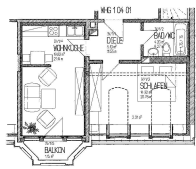
HUMBOLDTSTR. 21, DACHGESCHOSS, 2-RAUM-WOHNUNG NR. 10/0403 NEUBAU/MIETWEG/MIETWEG KASSEL/FRANKENBERG M 1:100
